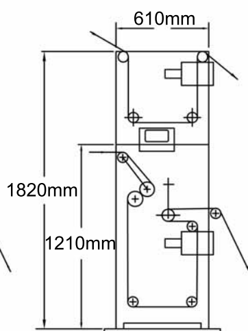
1 Alimentadora y 2 Guías de Banda
