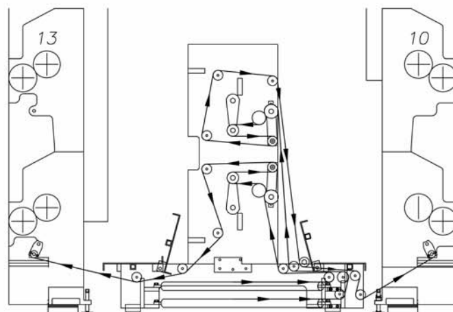
2 Alimentadoras entre torres
