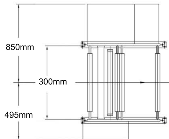
4 Alimentadoras y Guidas de Banda
