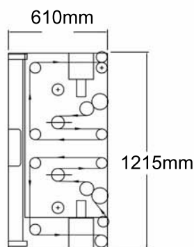
2 Alimentadoras y 2 Guías de Banda
